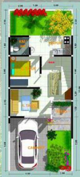
DENAH LANTAI BAWAH
